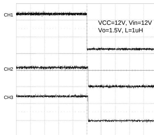
Shutdown (EN=GND)
